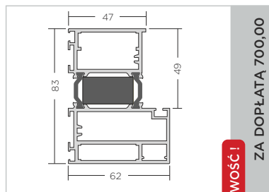
ościeżnica Termo ALU 68
