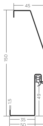
OŚCIEŻNICA PD68/150
