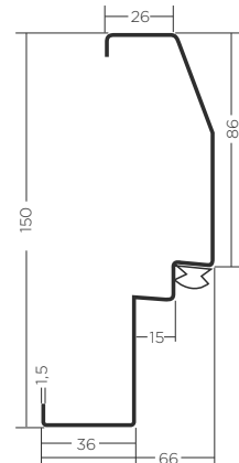
OŚCIEŻNICA PM84/150
