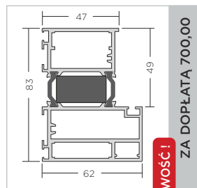
ościeżnica Termo ALU 68
