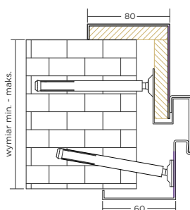
ościeżnica regulowana PU-PR z profilem sprzęgającym
