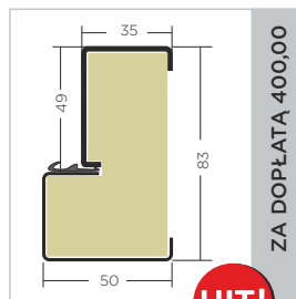
ościeżnica Termo ODS68
